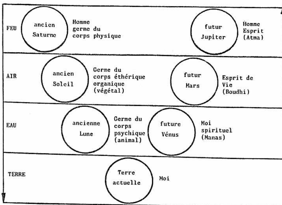
L'EVOLUTION DE LA TERRE
